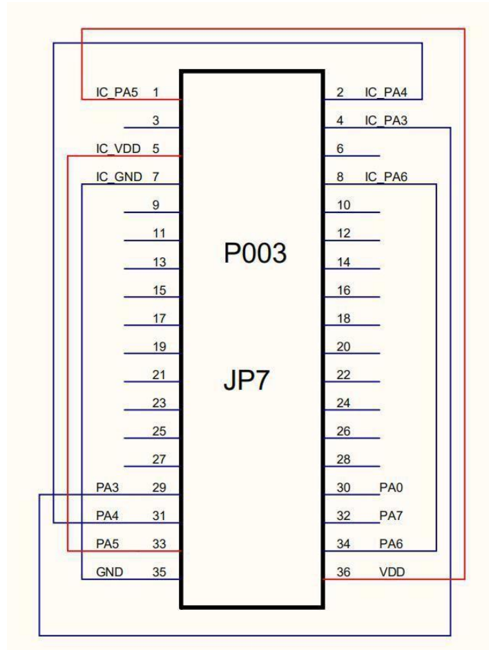
图 21: 使用 P003 时, P3608 (S08B) JP7 跳线原理图
