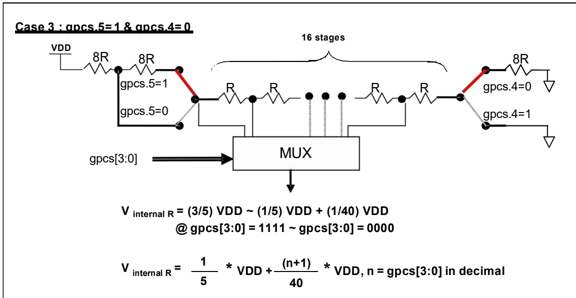
图 7: V_{\text{internal R}} 硬件接法 ( gpc5.5=1 & gpc5.4=0 )
