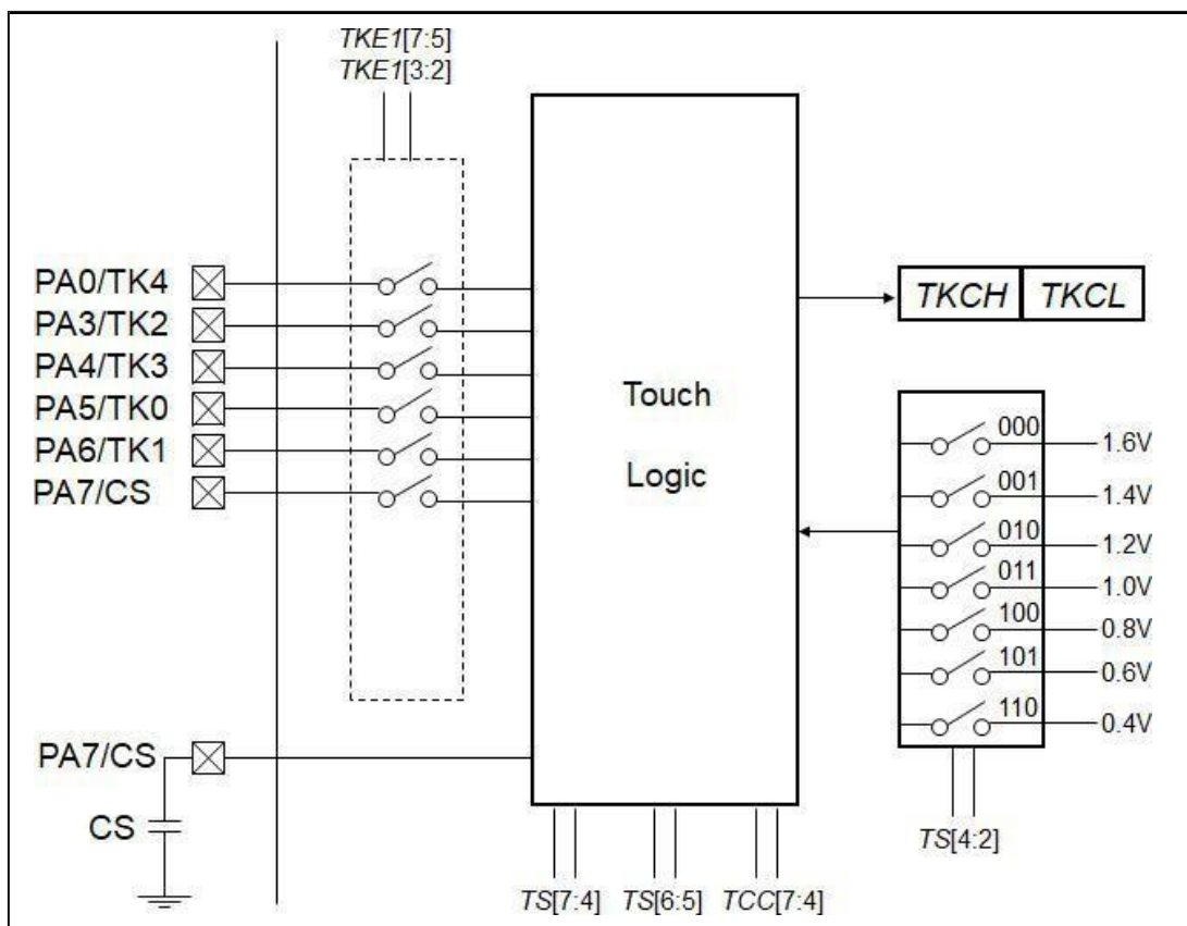
图 17: 触摸检测电路的功能方框图
