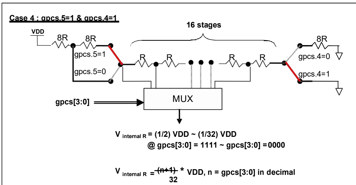
图 8: V_{\text{internal R}} 硬件接法 ( gpc5.5=1 & gpc5.4=1 )
