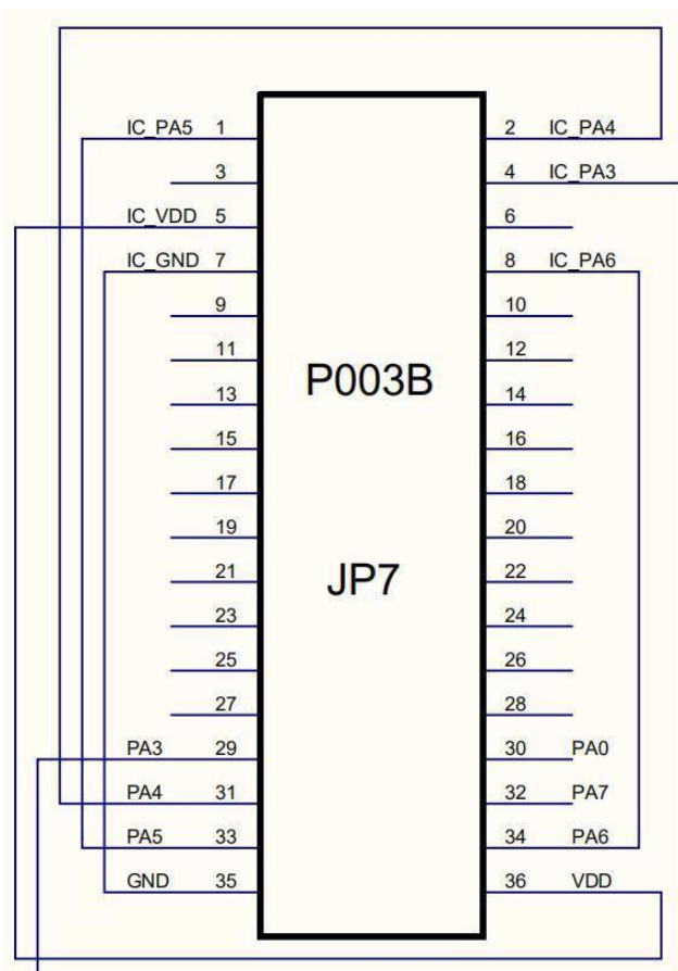
图 23: 使用 P003B 时, P3608 (S08B) JP7 跳线原理图
