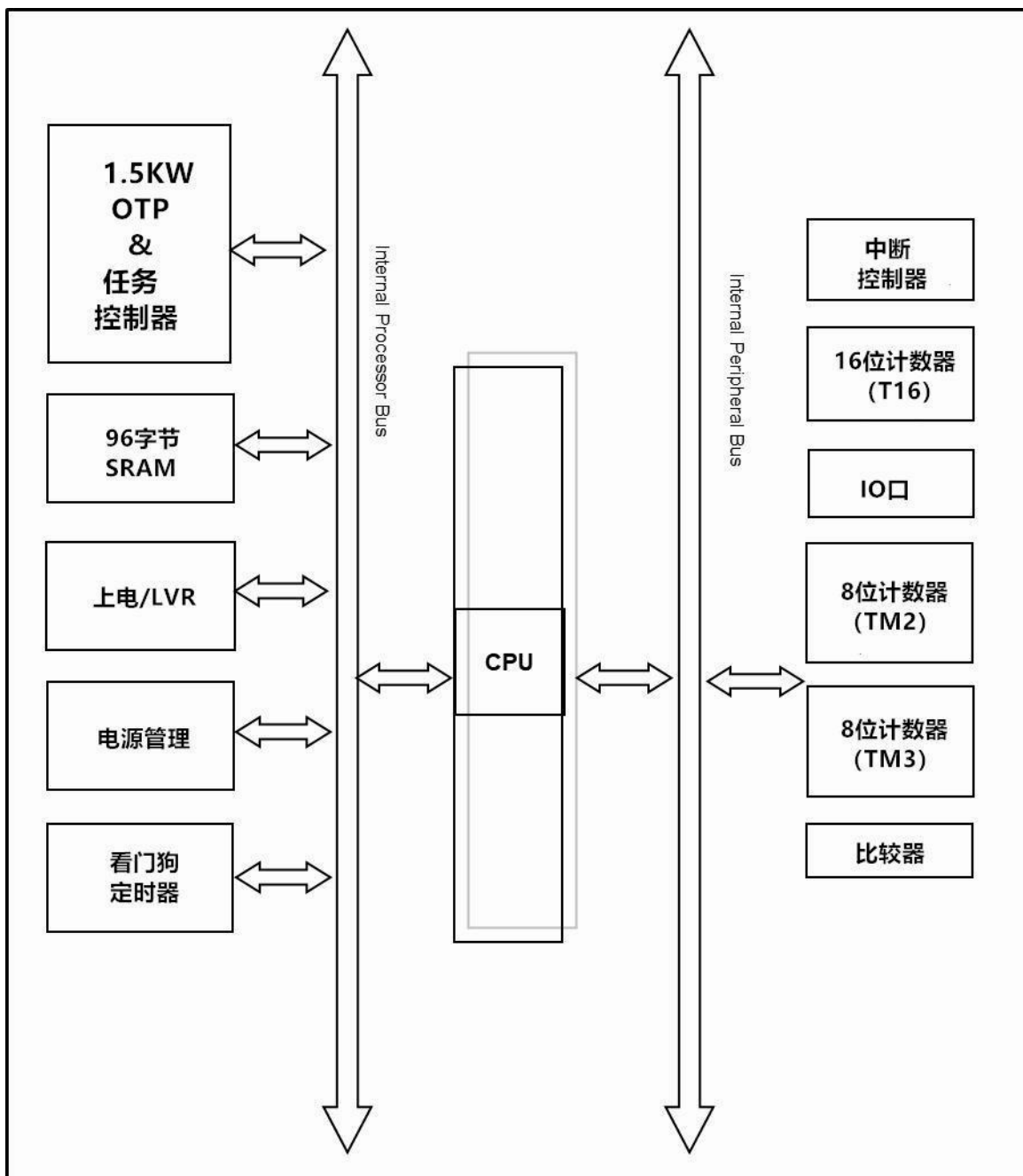
图 1: P36X系列系统方框图
