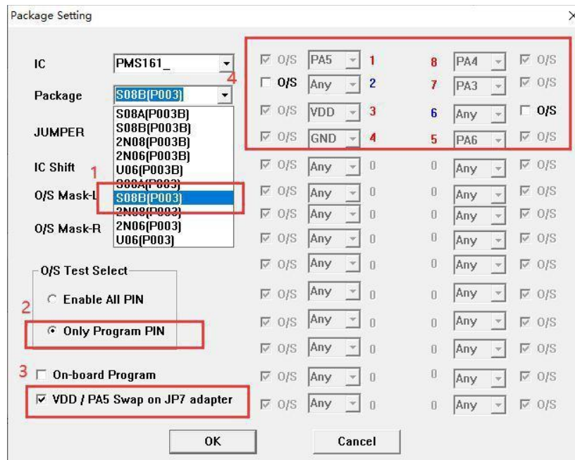
图 20: P308-S08B 在 P003 转档配置
