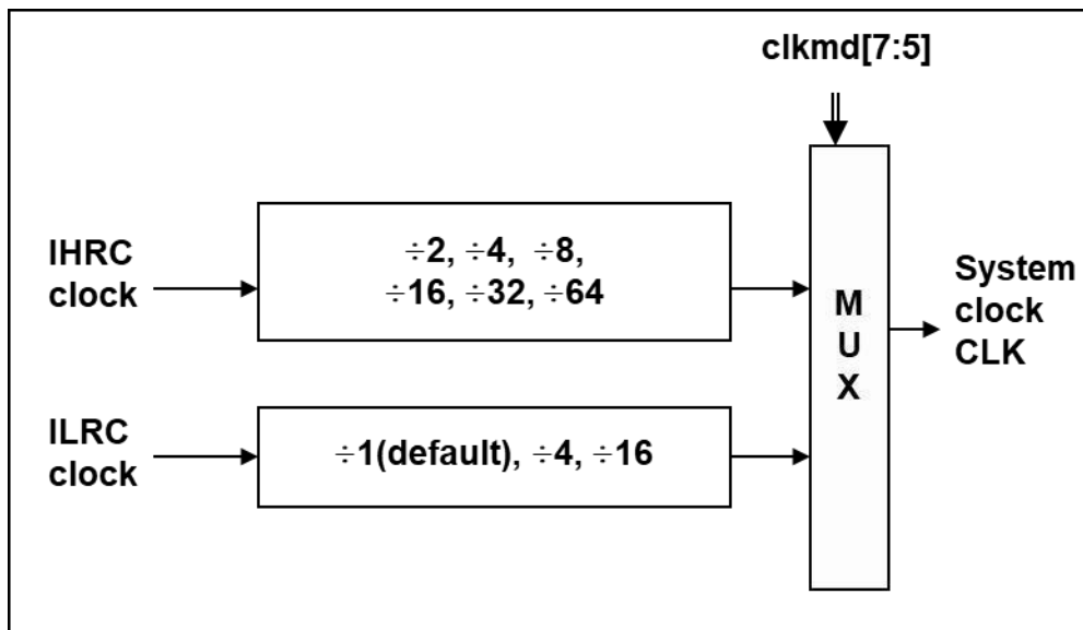
图 3: 系统时钟选项 使用者可以在不同的需求下选择不同的系统时
