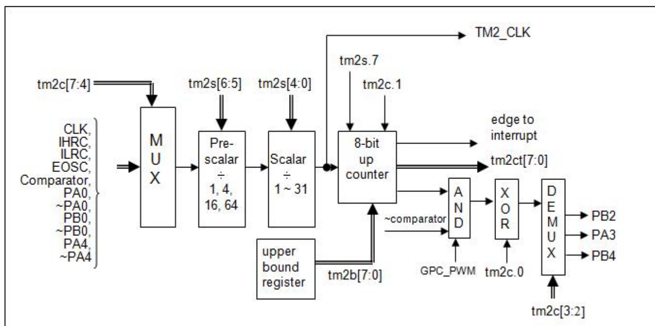
图 10: Timer2 硬件框图
