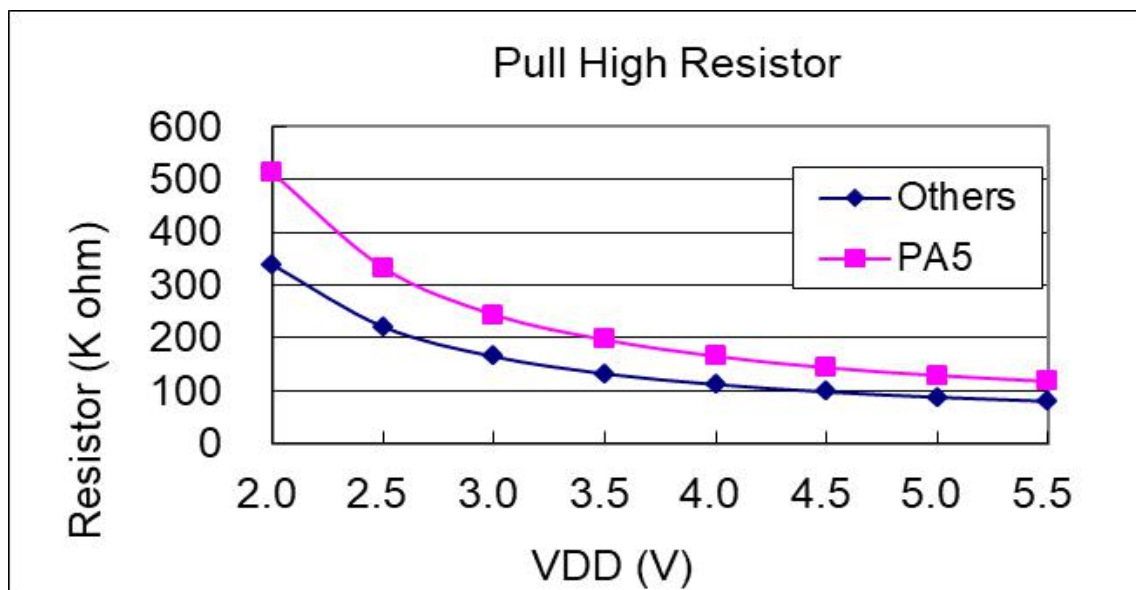
4.14. IO 引脚上拉阻抗曲线图
