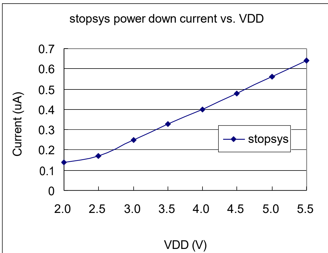
4.15. 掉电消耗电流( I_{PD} )与省电消耗电流( I_{PS} )关系曲线图
