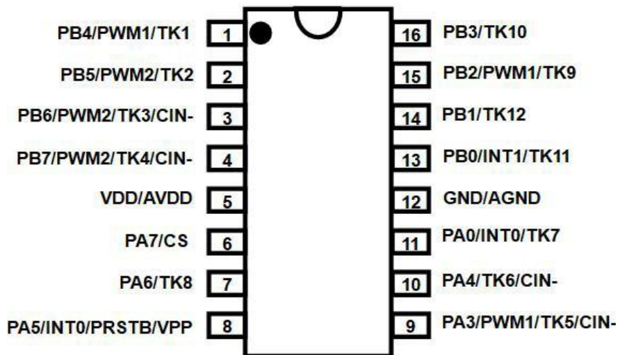
P3903: SOP16 (150mil)
