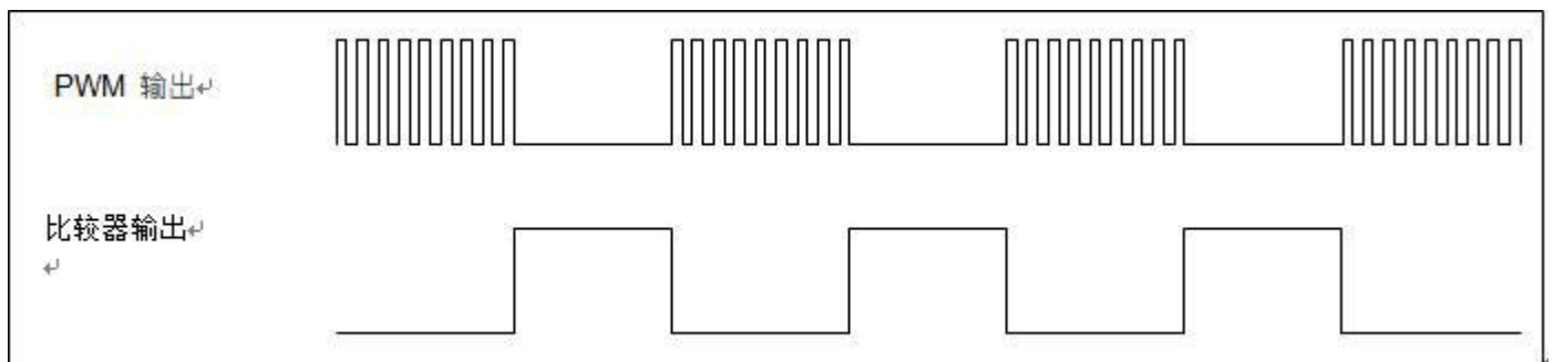
图 15: 比较器控制 PWM 输出
