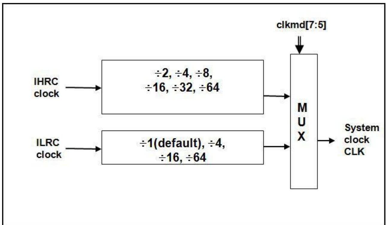
图 3: 系统时钟选项 使用者可以在不同的需求下选择不同的系统时钟, 选定的
