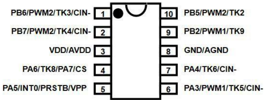
P3910: ESSOP10 (150mil) B
