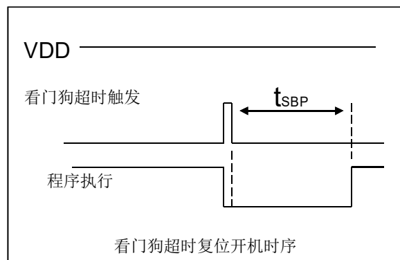
图 10: 看门狗超时溢出时序图
