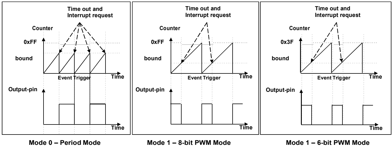
图 14: Timer2 周期模式和 PWM 模式的时序图(tm2c.1=1)
