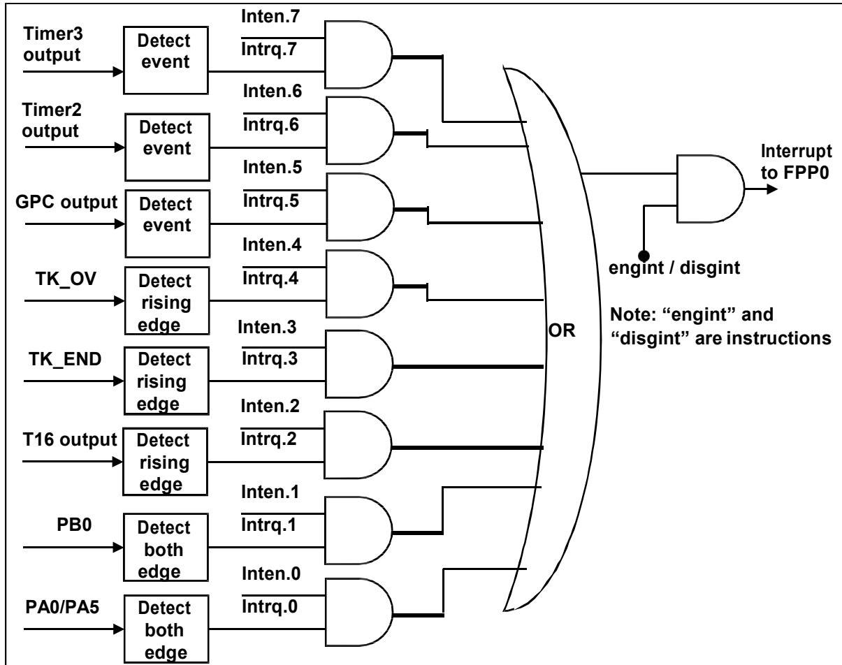
图 11: 中断控制器硬件框
