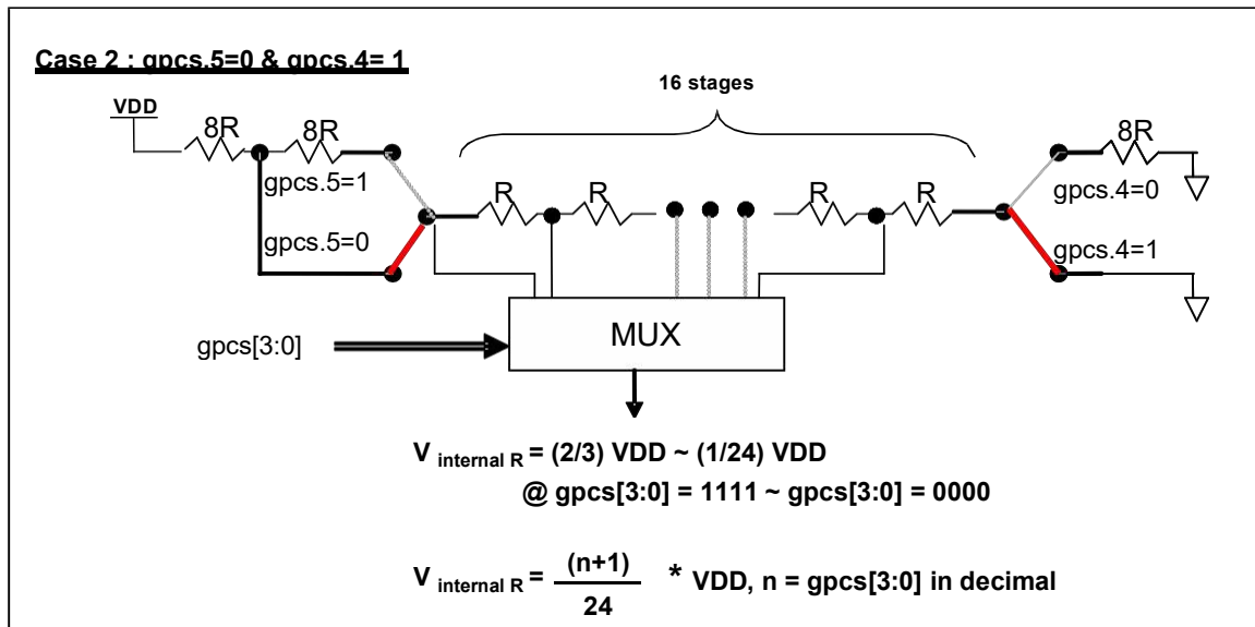
图 6: V_{\text{internal R}} 硬件接法 (gpcs.5=1 & gpcs.4=1)
