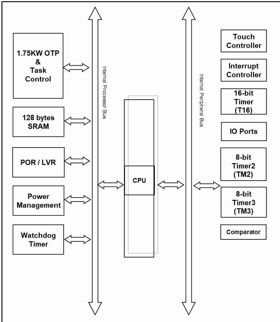
图 1: P39X系列系统方框图
