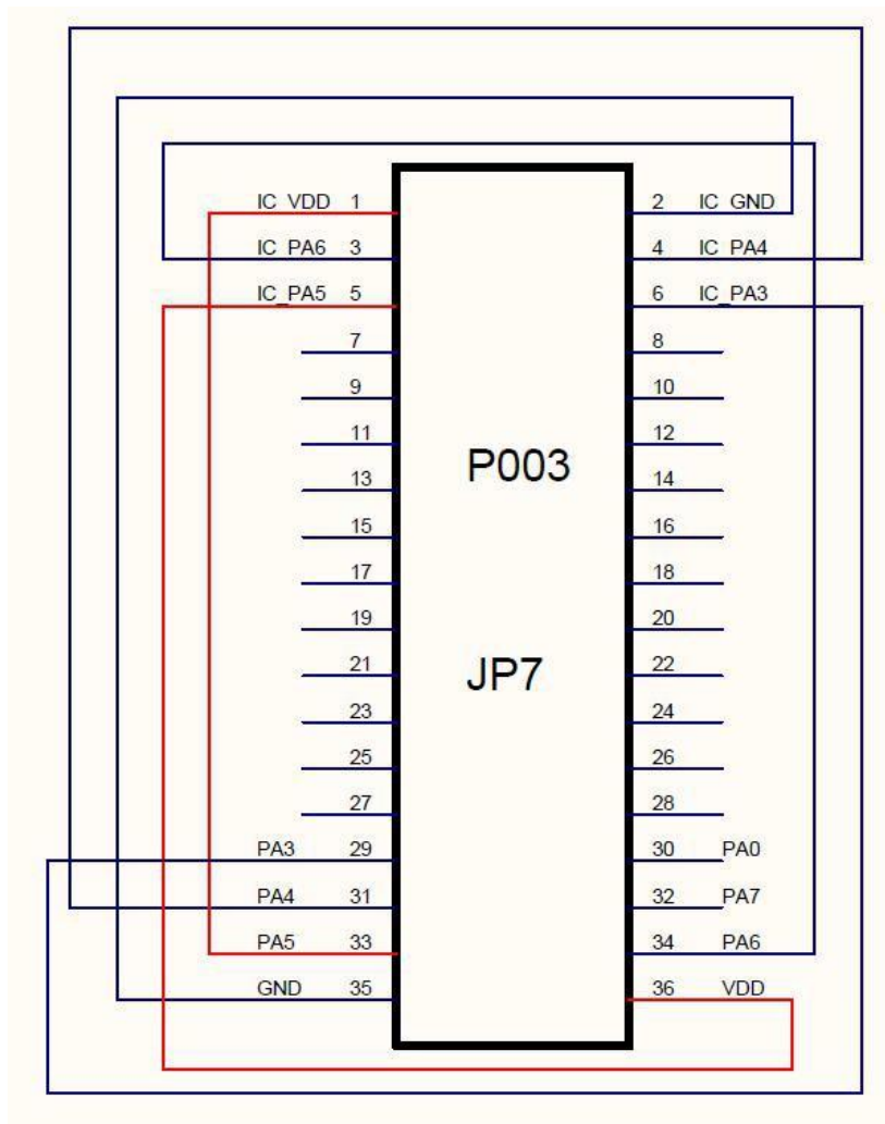
图 27：使用 P003 时，P33X 系列-S0P8 JP7 跳线原理图
