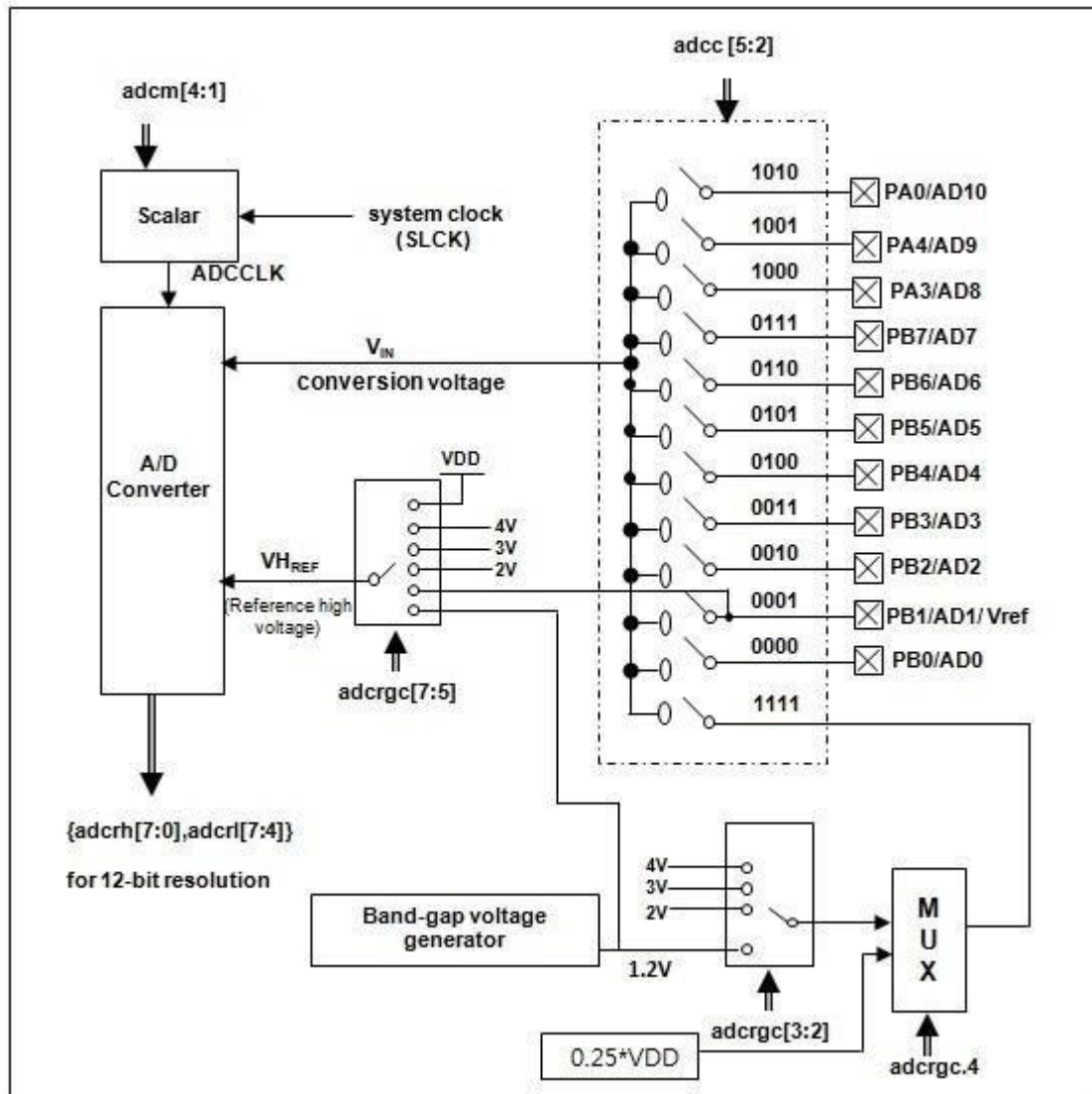
图 22: ADC 模块框图当使用 ADC 模块时有 7 个寄存器需要配置, 它们是:
