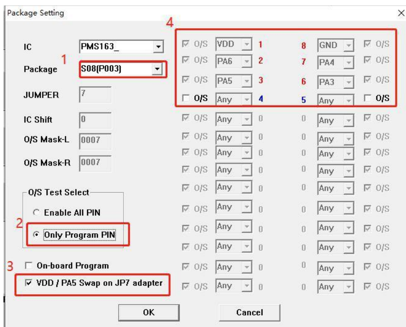
图 26: P33X 系列-S0P8 在 P003 转档配置
