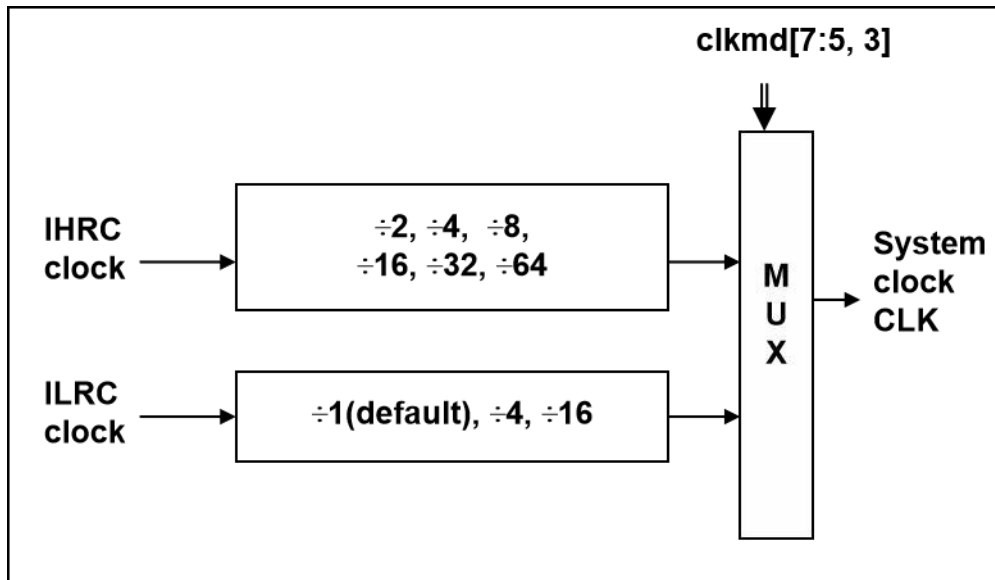
图 3: 系统时钟选项 使用者可以在不同的需求下选择不同的系统时钟, 选定的系统时钟应与电源电压和 LVR 的基准位结合起来才能使系统稳定。LVR 的基准位是在编译过程中选择, 不同系统时钟对应的 LVR 设定, 请参考章节 4.1 中系统时钟的最低工作 电压。
