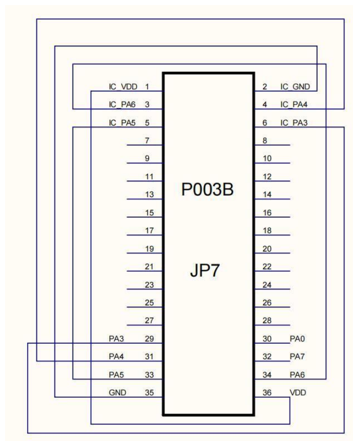
图 29: 使用 P003B 时, PP33X 系列-S0P8 JP7 跳线原理图
