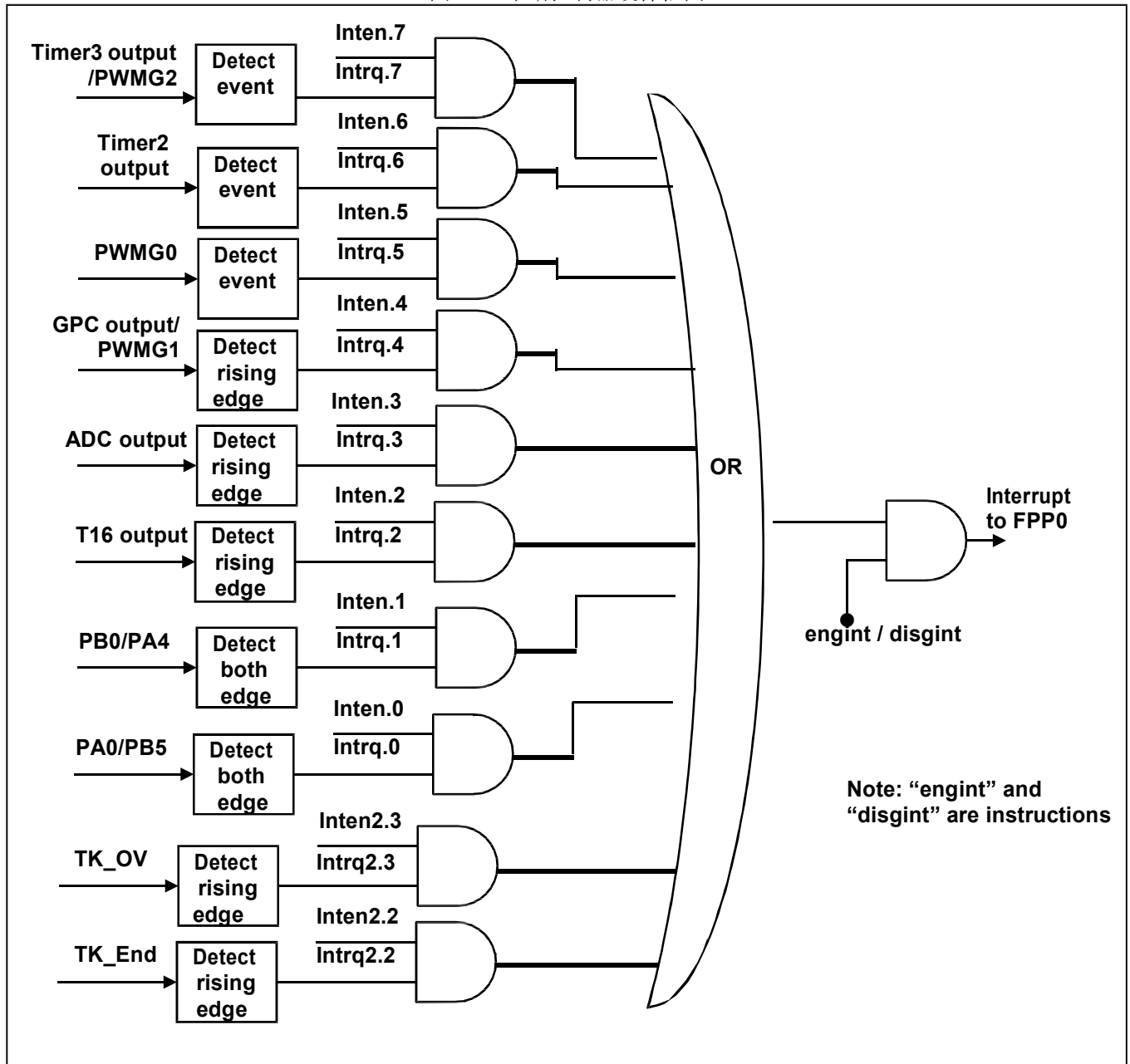
图 11：中断控制器硬件框图
