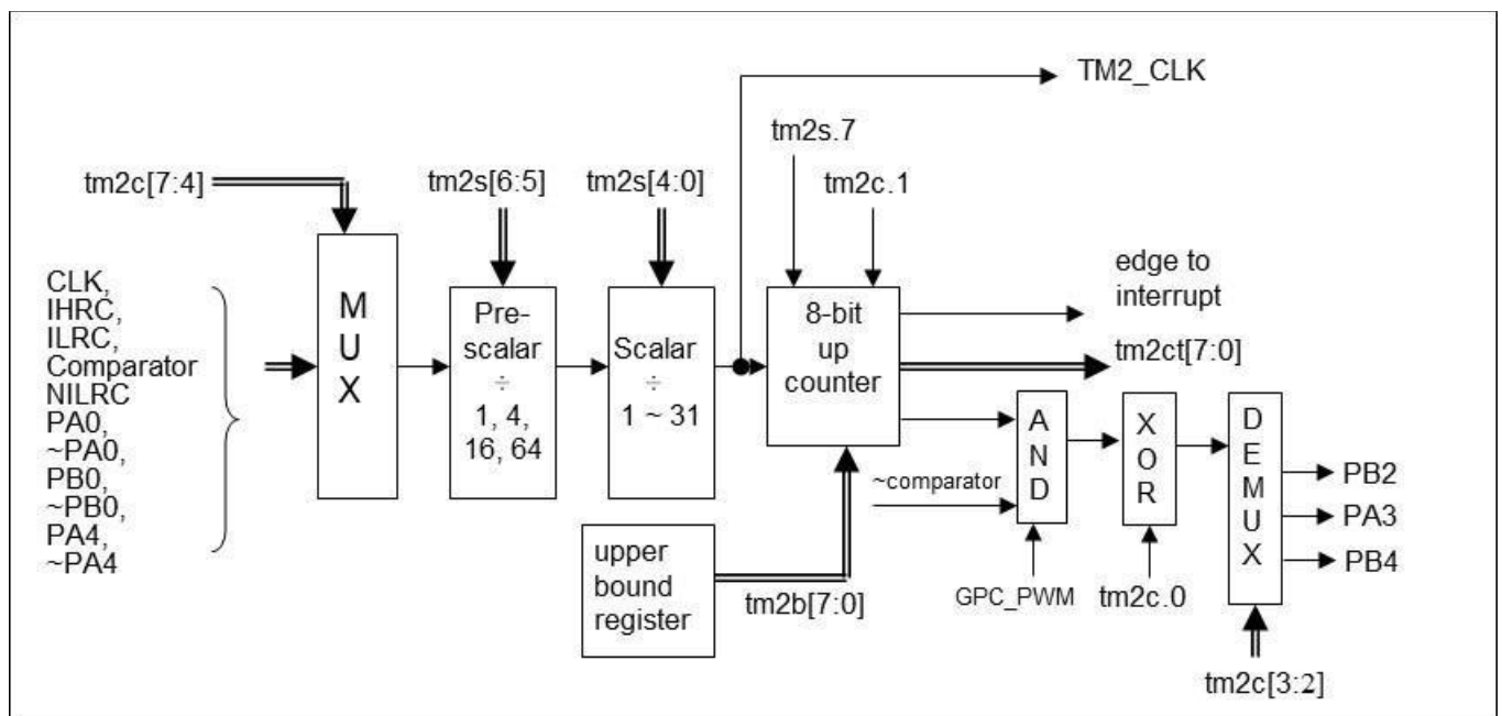
图 13: Timer2 硬件框图
