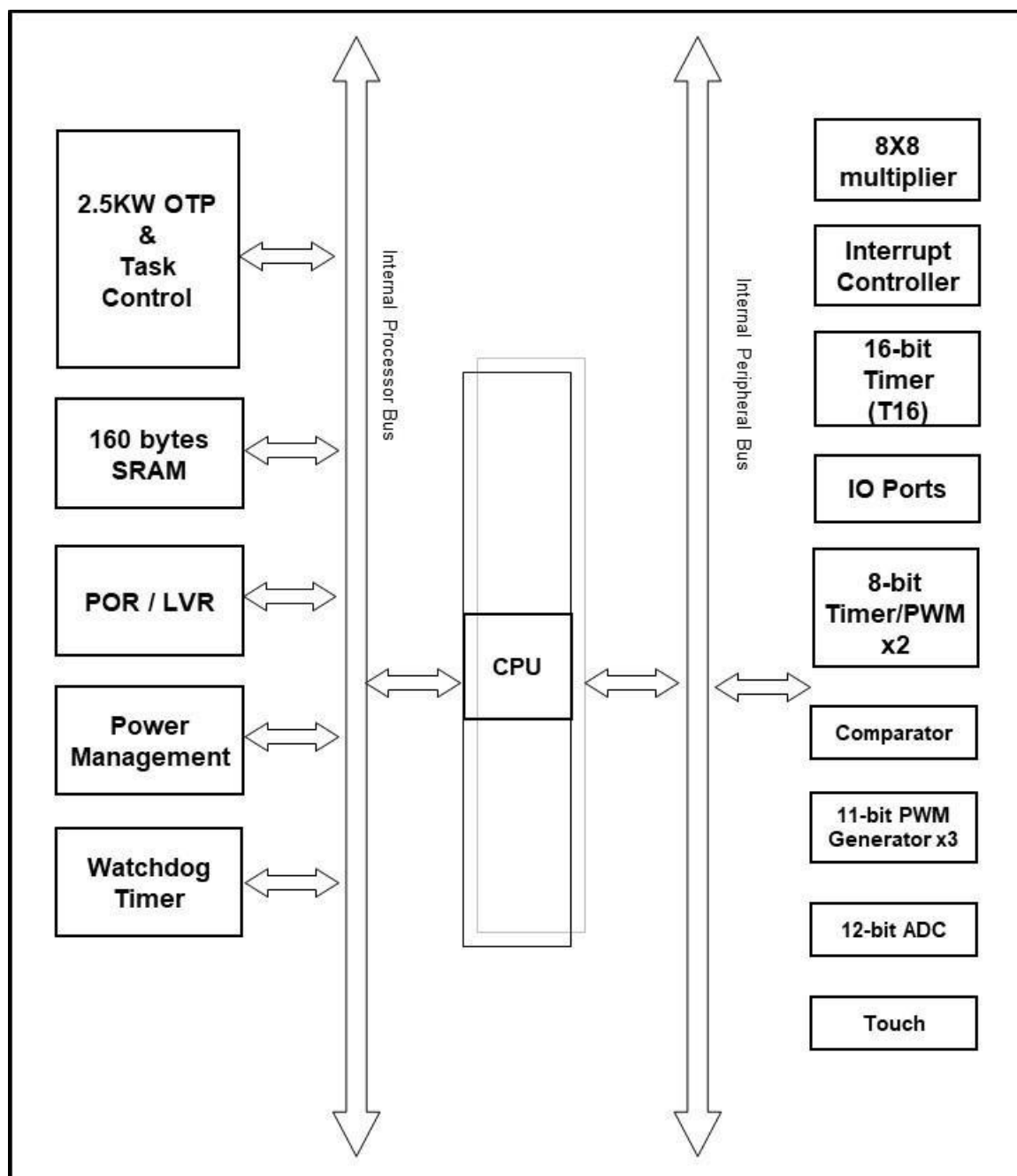
图 1：P33X 系列系统方框图
