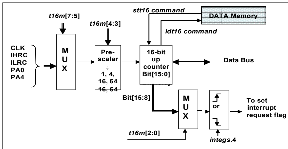
图 9: Timer16 模块框图
